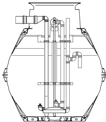
Querschnitt Beleb-ung
